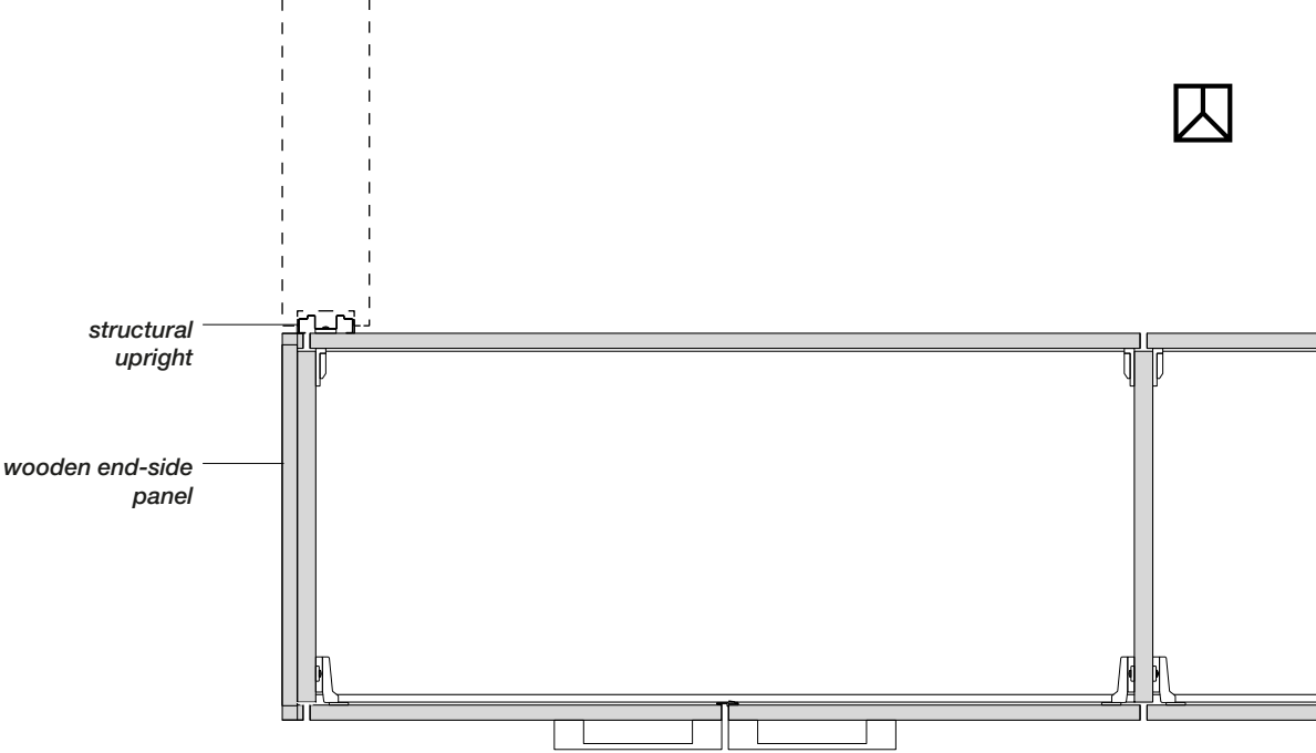
90° corner Quadra- to- Metrica Structural
