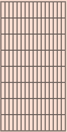
03 - Fresatura verticale 04 - Fresatura orizzontale 1088x2176x12 mm
