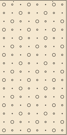
Echo 01 - 1088x2176x12mm 02 - 1088x2720x12 mm
