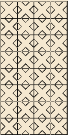
Diamond 01 - 1088x2176x24 mm 02 - 1088x2720x24 mm
