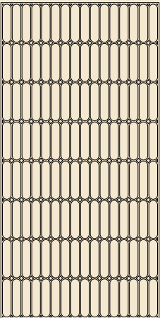
Capsule 01 - 1088x2176x24 mm 02 - 1088x2720x24 mm
